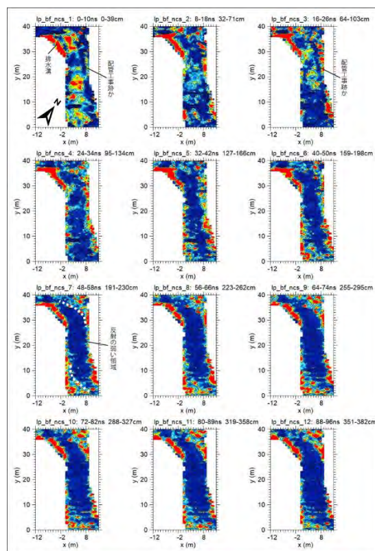
図 2 地中レーダー探査成果図
