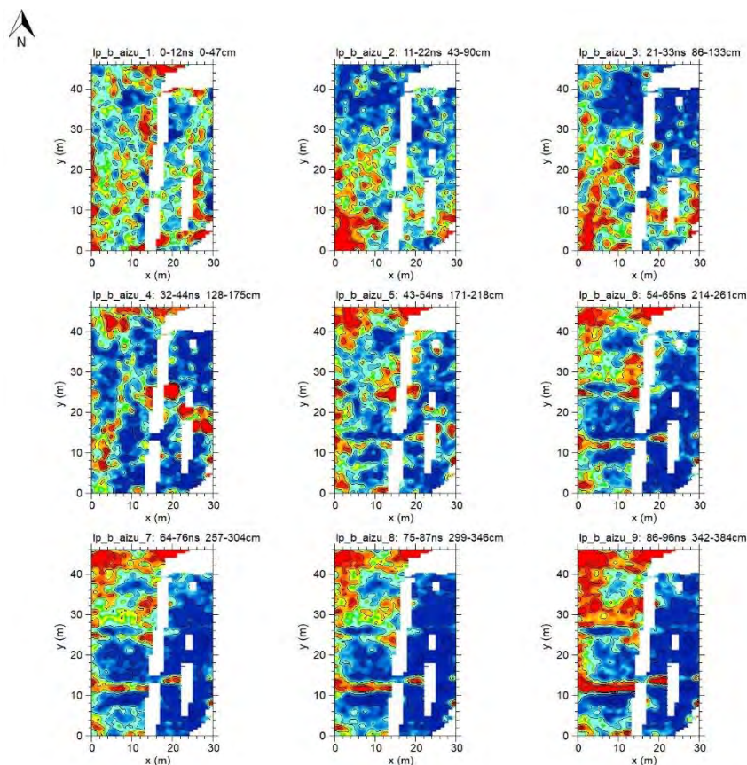
図 1 地中レーダー探査の結果
