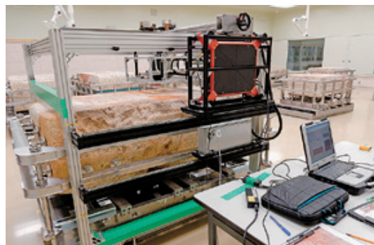
テラヘルツ分光法による粗鬆化した漆喰部分の検出のテスト施行 (東京文化財研究所)
