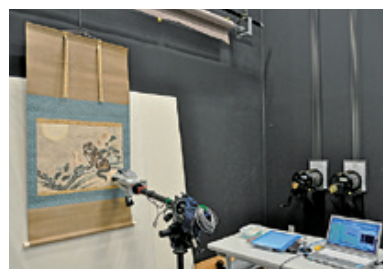
可搬型蛍光X線分析装置を用いた絵画の彩色材料調査
